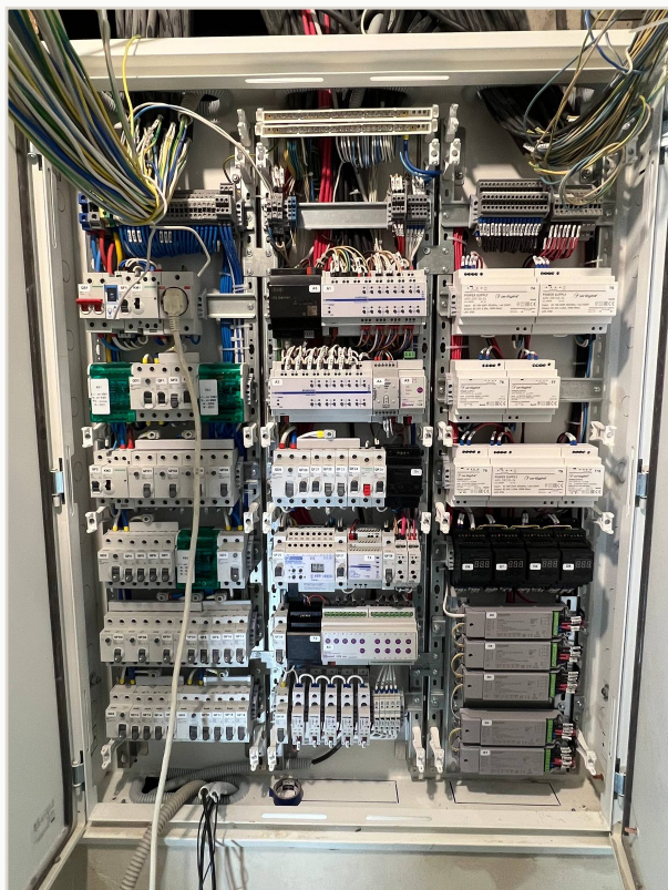
Сборка щита автоматики
